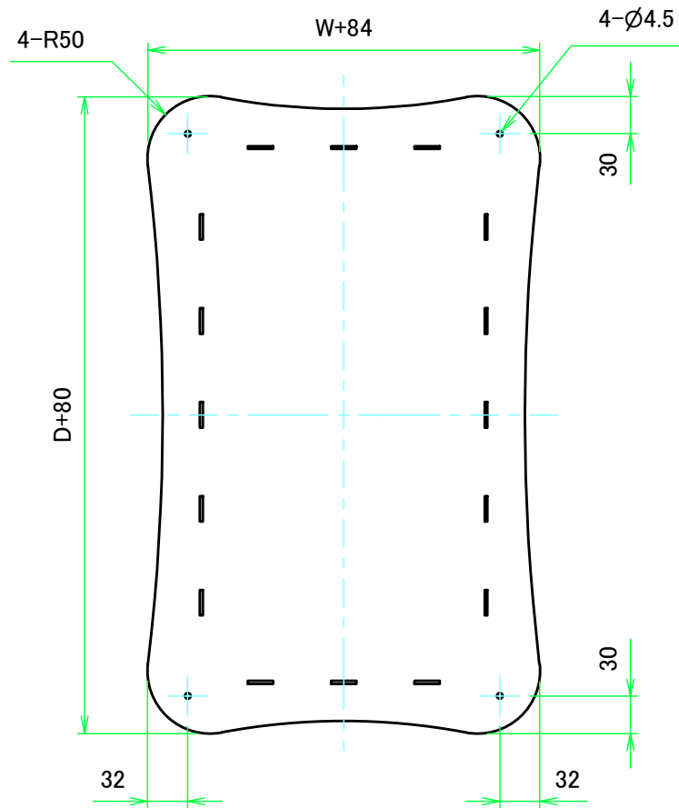
上カバー表面 / Top cover Frontside
